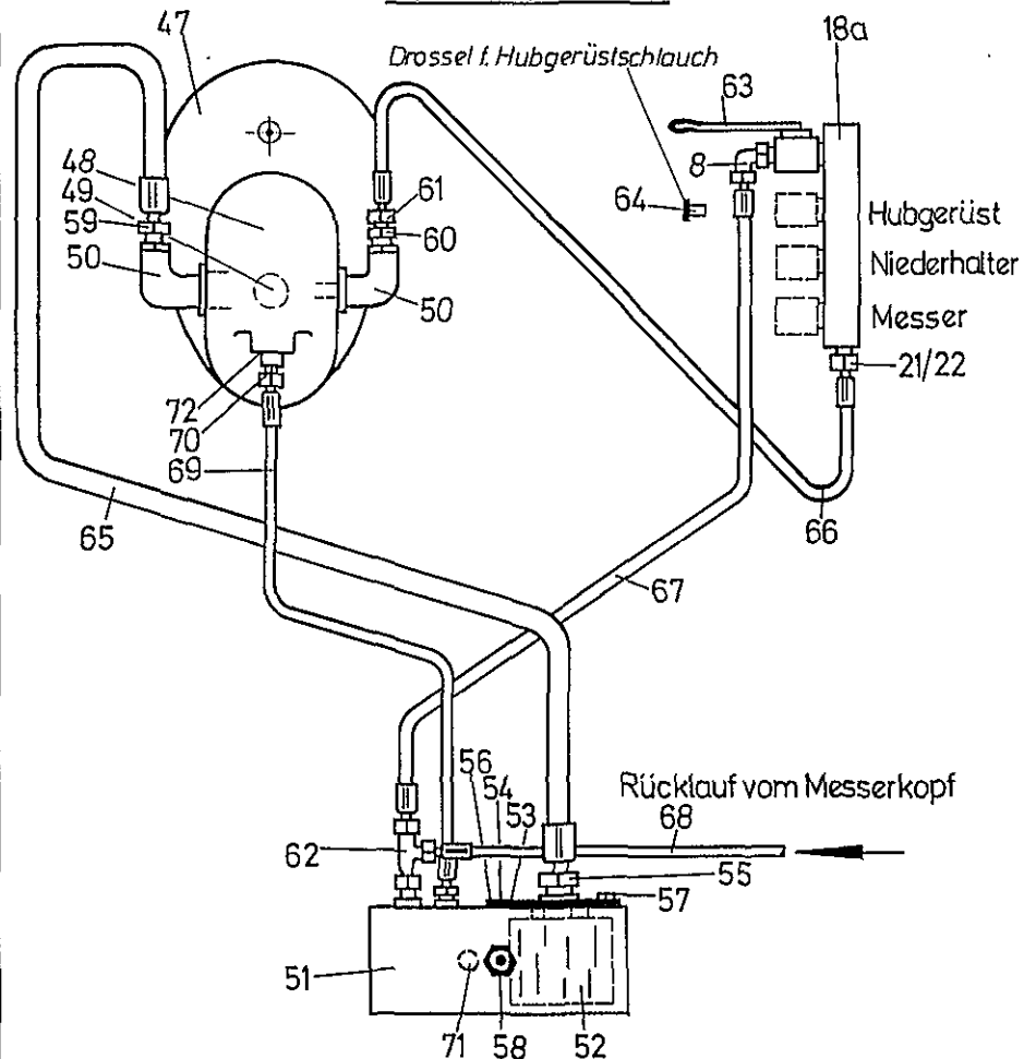
Anschlußplan IV Hydr. Pumpenanlage
