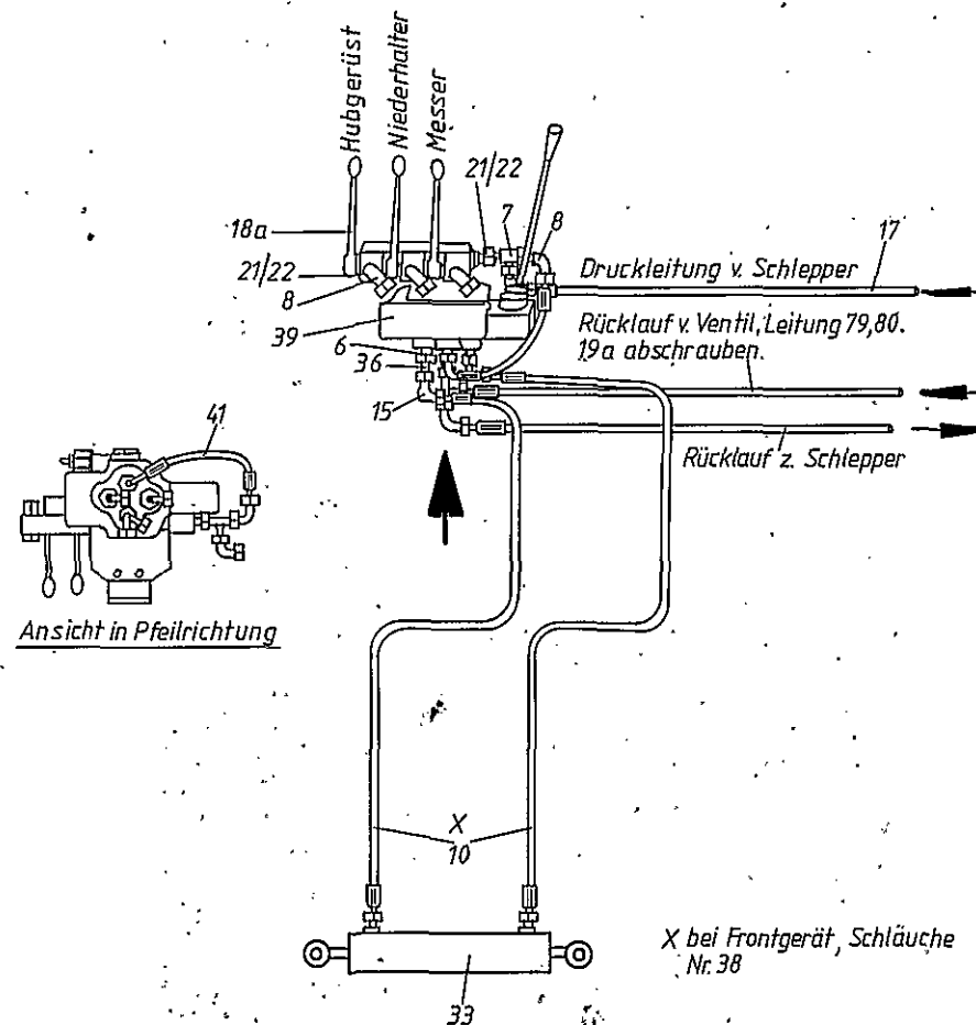
Anschlußplan II Für hydr. Oberlenker mit Steuergerät
