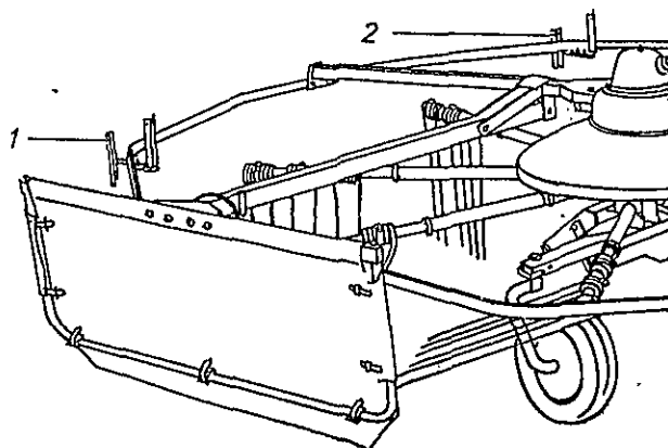
Montage Beleuchtungshalter
